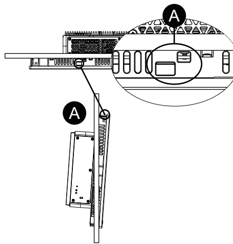
A. 낙하 방지 잠금장치
