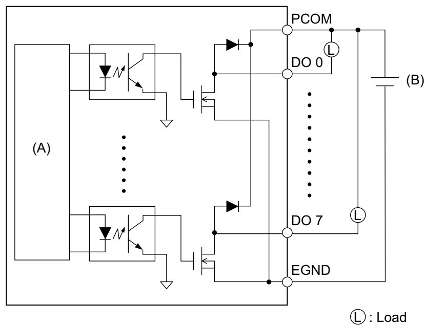
(A) 内部电路
