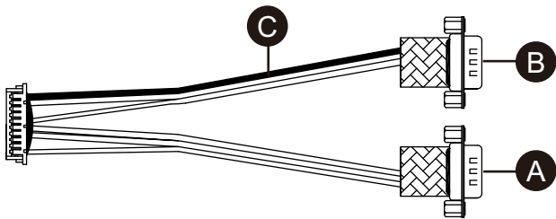
RS-422 インターフェイスクーブル
