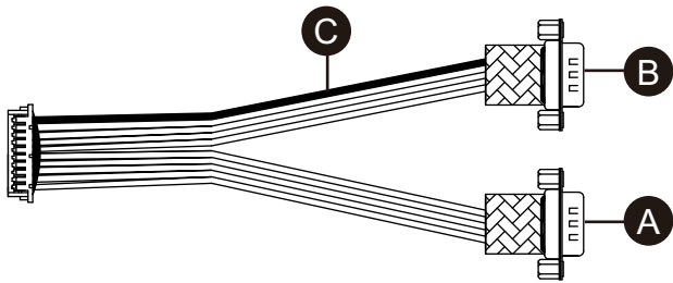
RS-422 インターフェイスクーブル
