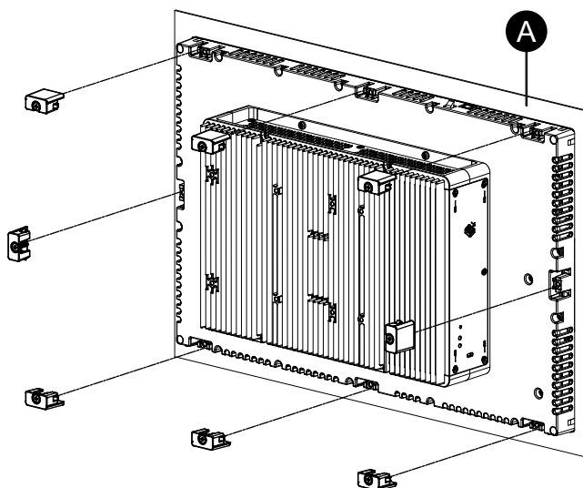
A. Schalttafel
