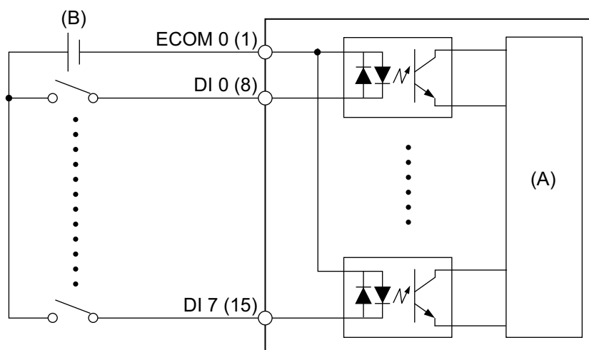
数字输入电路 (湿接点)
