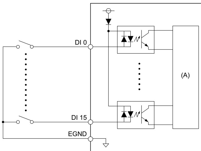
数字输入电路 (干接点)
