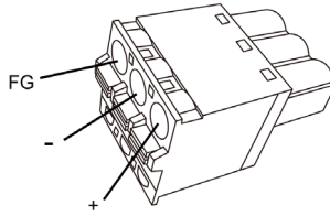
Gerader Stecker
