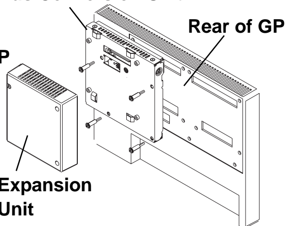
GP-2500
