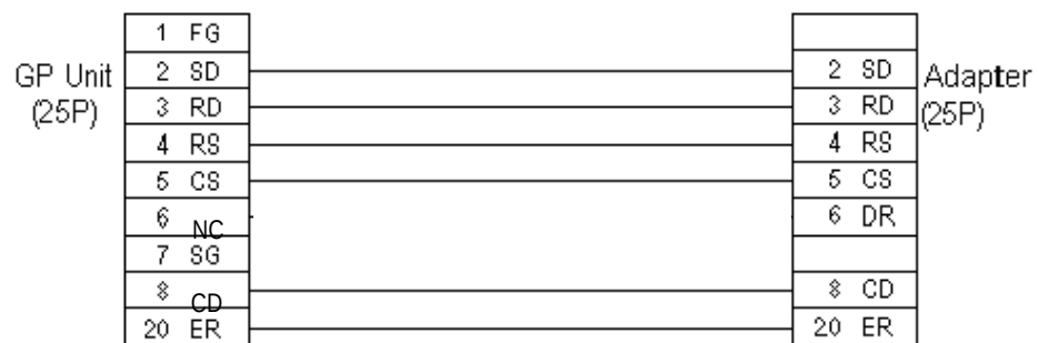
Cable Diagram 4 (RS-232C)
