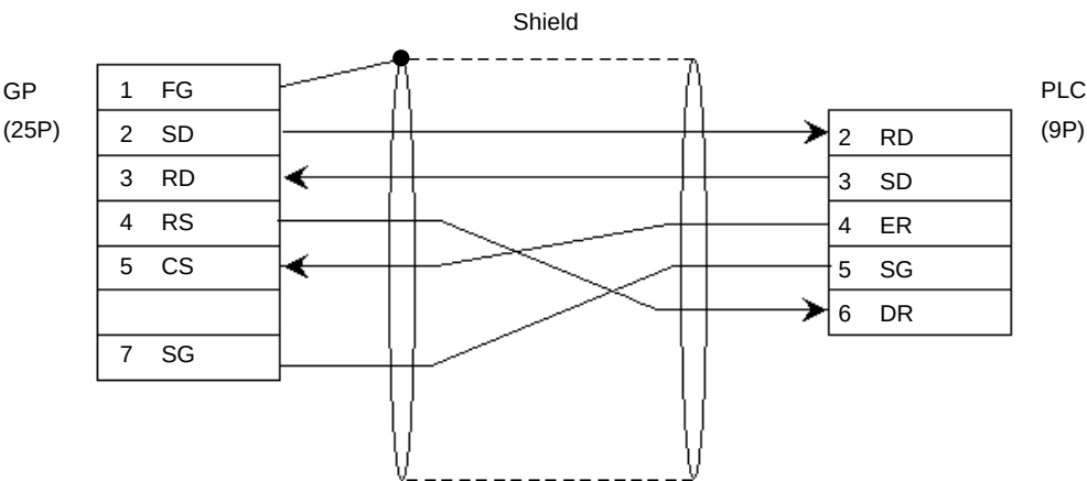
Cable Diagram 6 (RS-232C)
