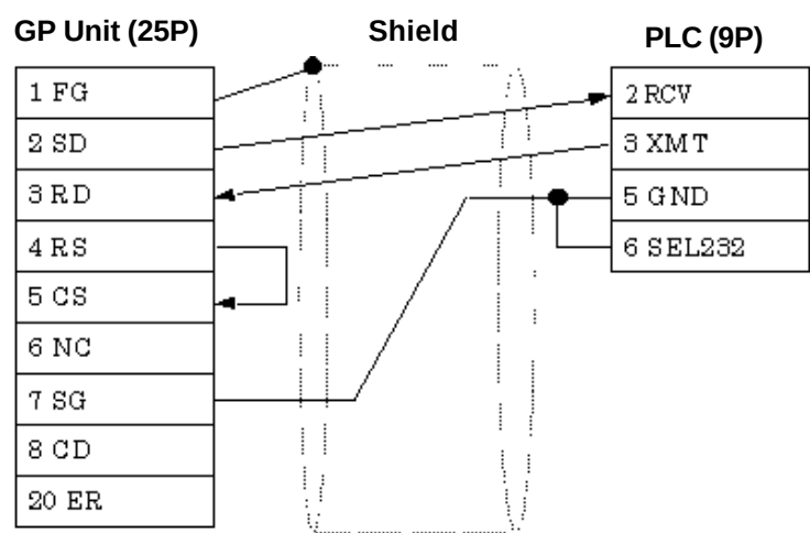
Cable Diagram 9 (RS-232C)
