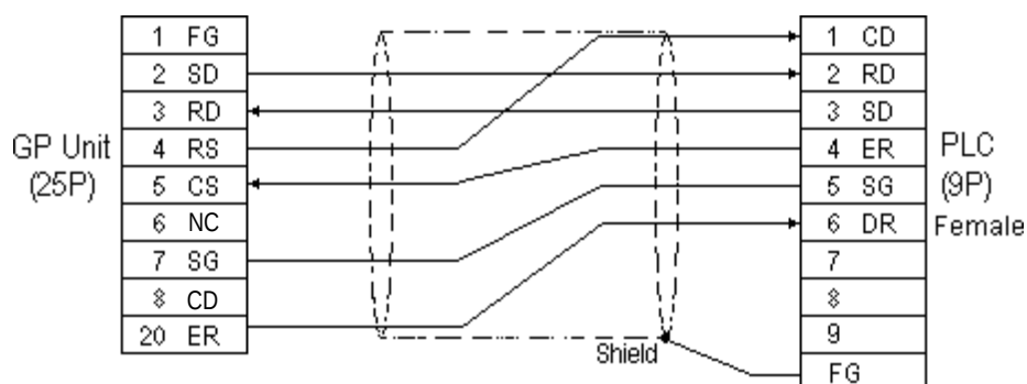
Cable Diagram 4 (RS-232C)
