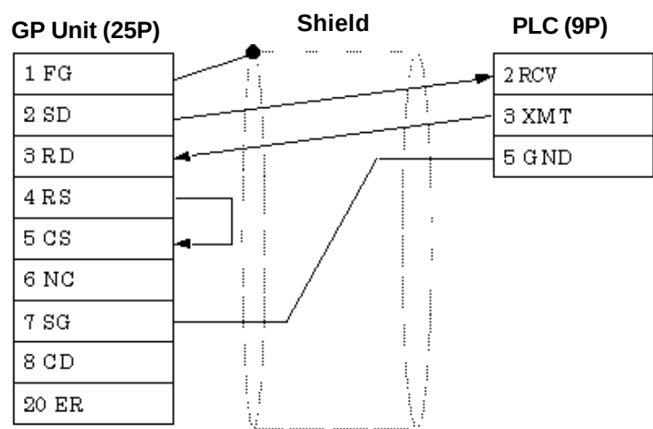
Cable Diagram 10 (RS-232C)
