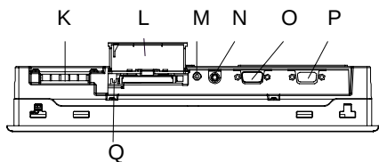
底面図
