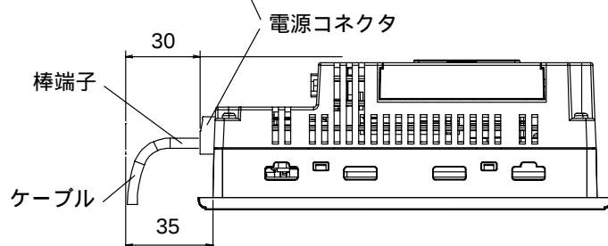
底面図
